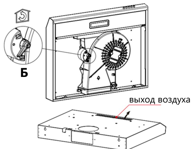
Режим рециркуляции (воздух проходит через угольный фильтр и возвращается в помещение)
