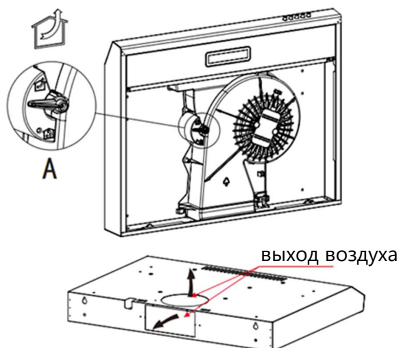
Вытяжной режим (отвод воздуха в вентиляцию)
