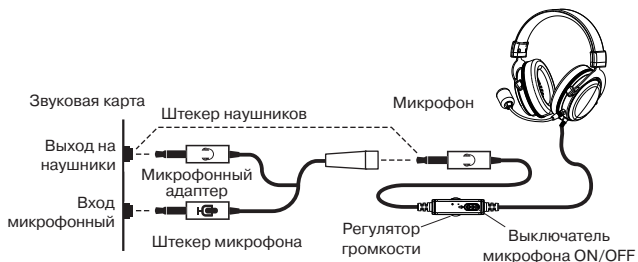
Рис. 2. Схема подключения
