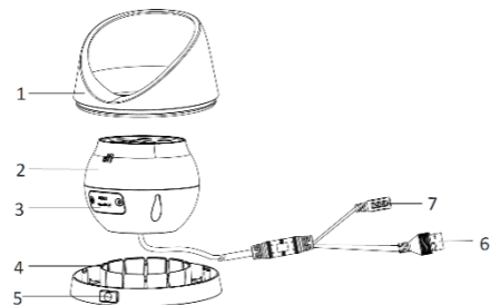
Рисунок 1-5 Купольная камера V типа
