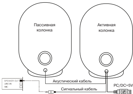
Рис. 2. Схема подключения
