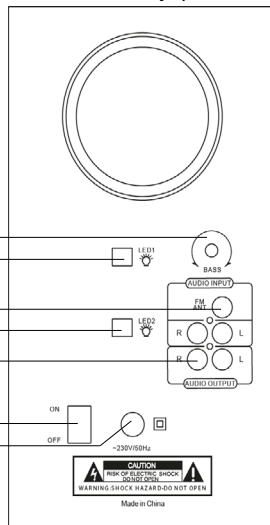
Мал. 2. Задня панель сабвуфера
