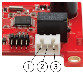
Низковольтное реле (базовая комплектация)
