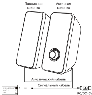
Рис. 2. Схема подключения
